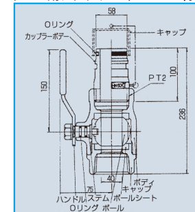
ワンタッチカップリング HK-50C(ボールバルブ付)
