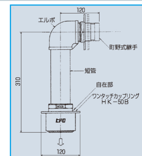
ホース用アダプター(HK-50B付)
