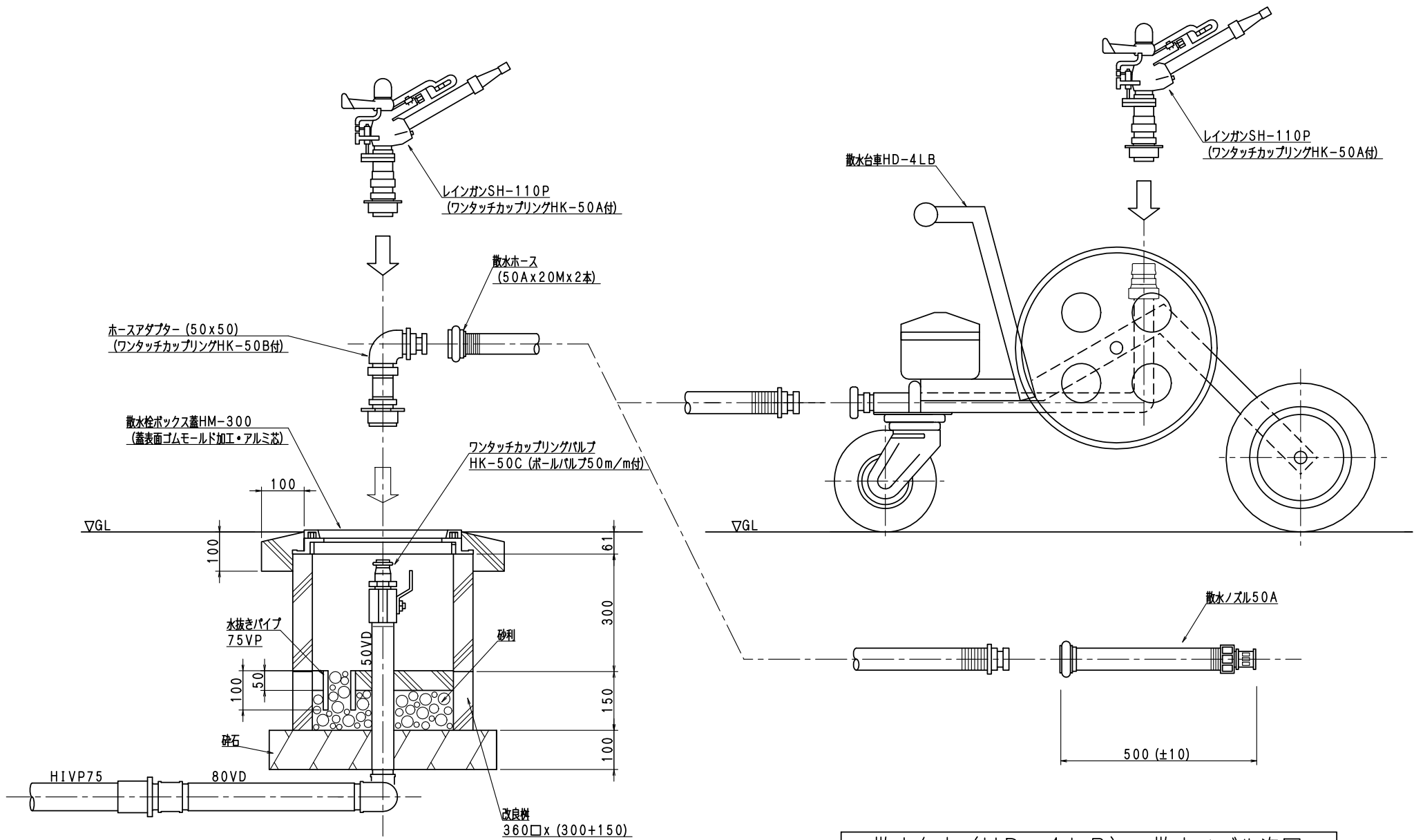
散水台車 (HD-4LB) ・散水ノズル姿図
