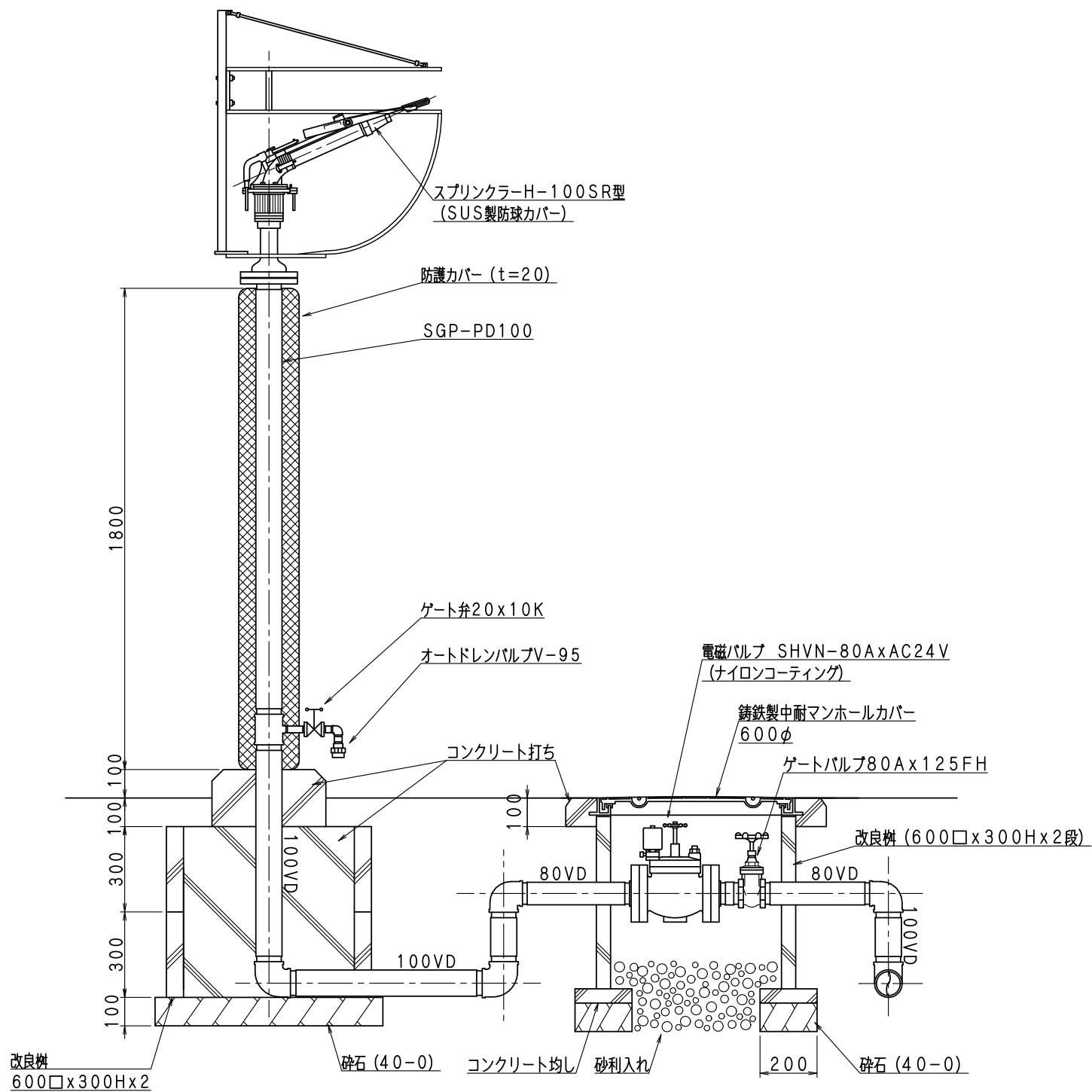
レインガン (H-100SR型) ・電磁弁 (SHVN-80) 装置取付詳細図
